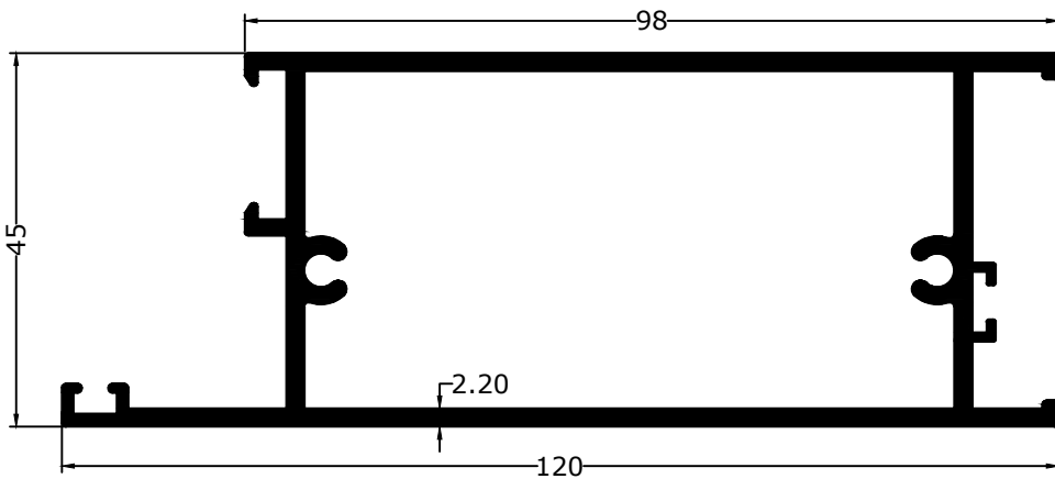
2281 2.032 KG/M
