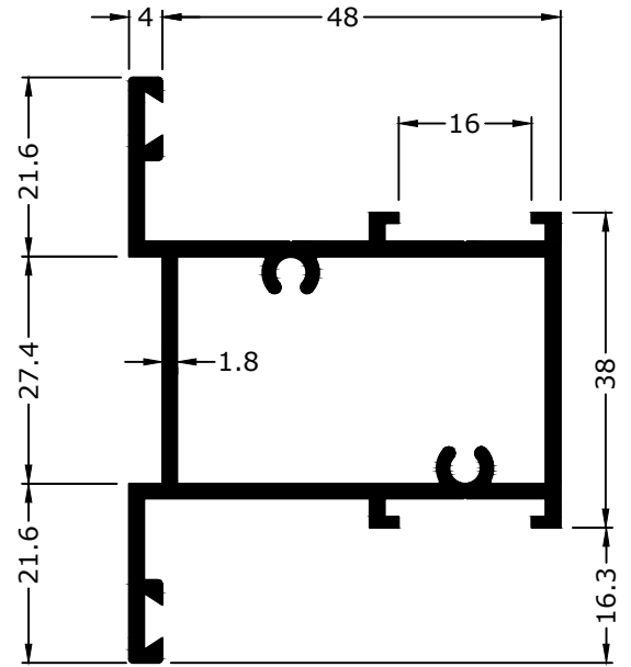
2056 1.187 KG/M
