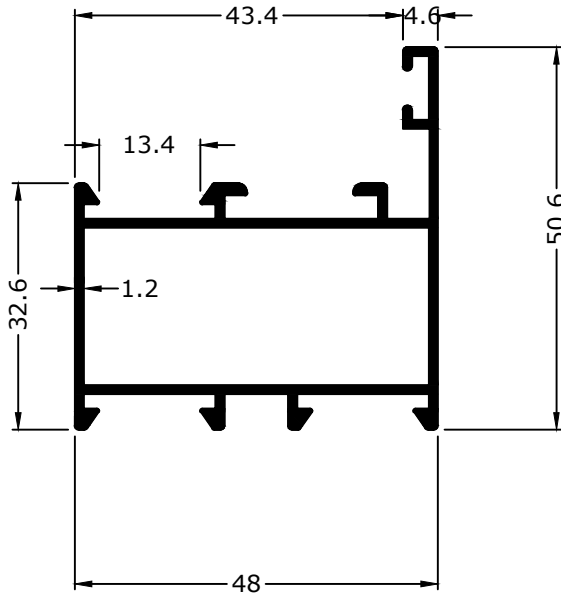
2071 0.737 KG/M
