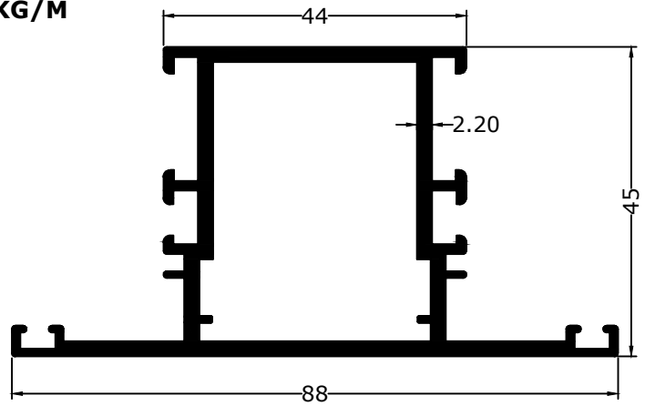
2251 1.457 KG/M
