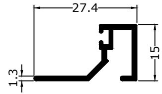
1510 0.216 KG/M
