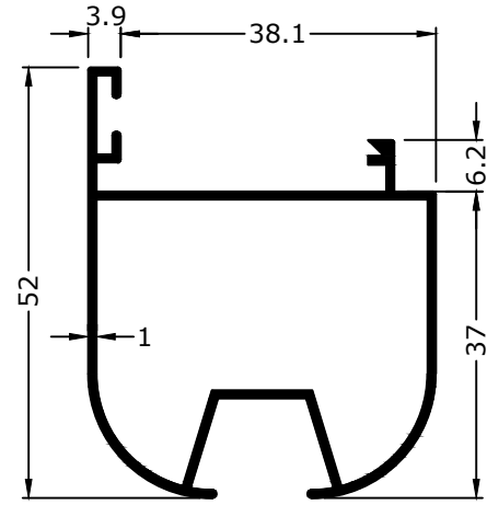
2067 0.545 KG/M
