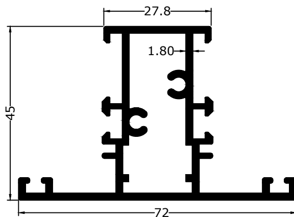
22332 1.260KG/M
