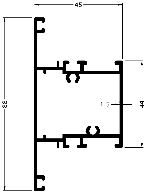
1732 1.204 KG/M
