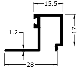
1032 0.256 KG/M
