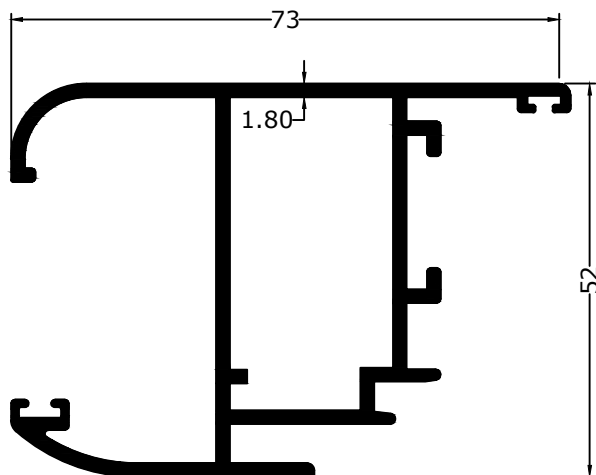
22322 1.325KG/M
