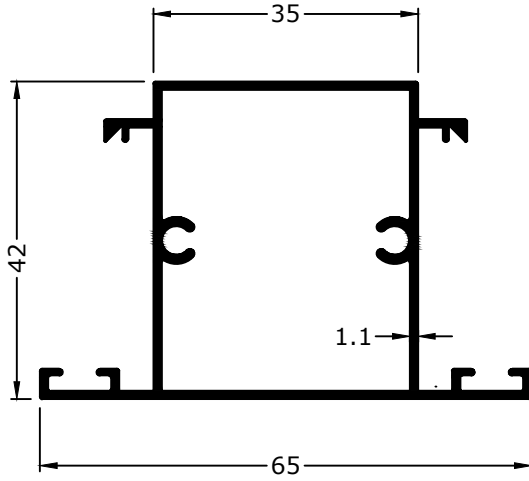
2999 0.706 KG/M
