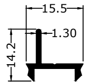
1157 0.108 KG/M
