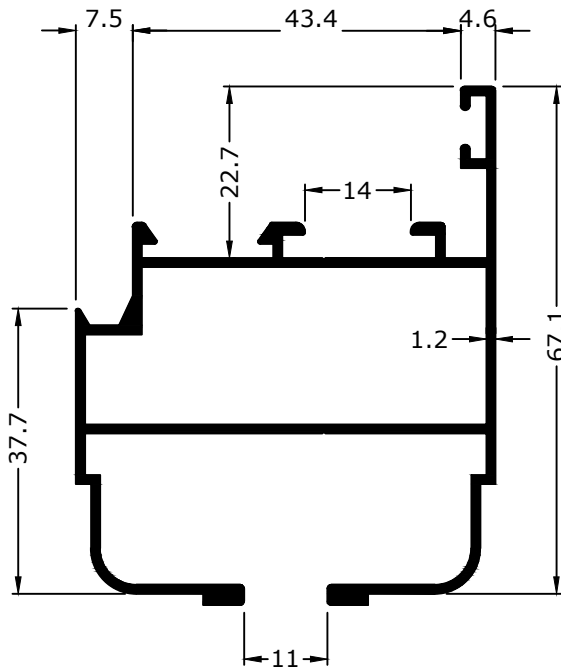
2073 1.005 KG/M
