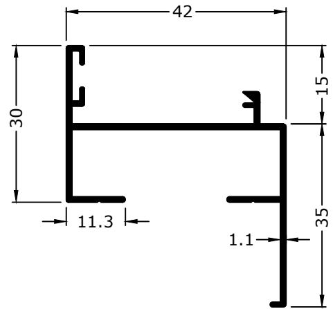
1016 0.426 KG/M
