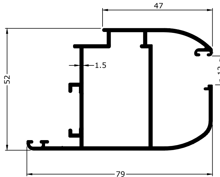
1729 1.200 KG/M
