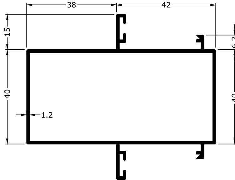
2040 0.987 KG/M
