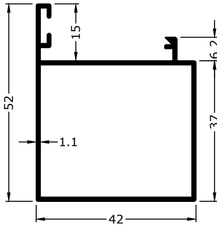
2068 0.560 KG/M
