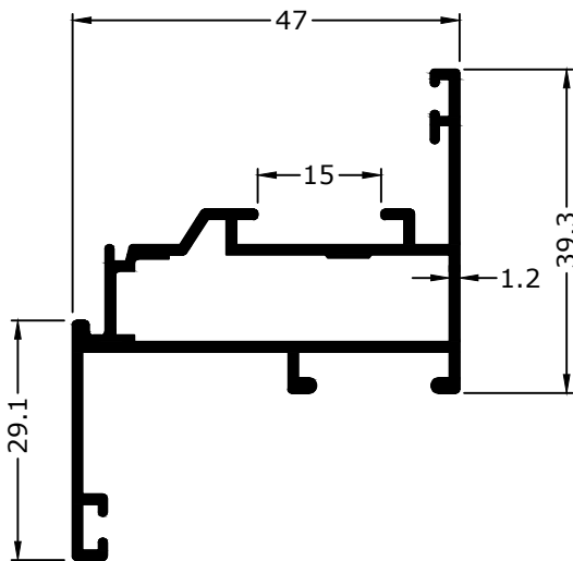
2138 0.702 KG/M
