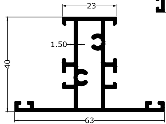
2211 0.938 KG/M
