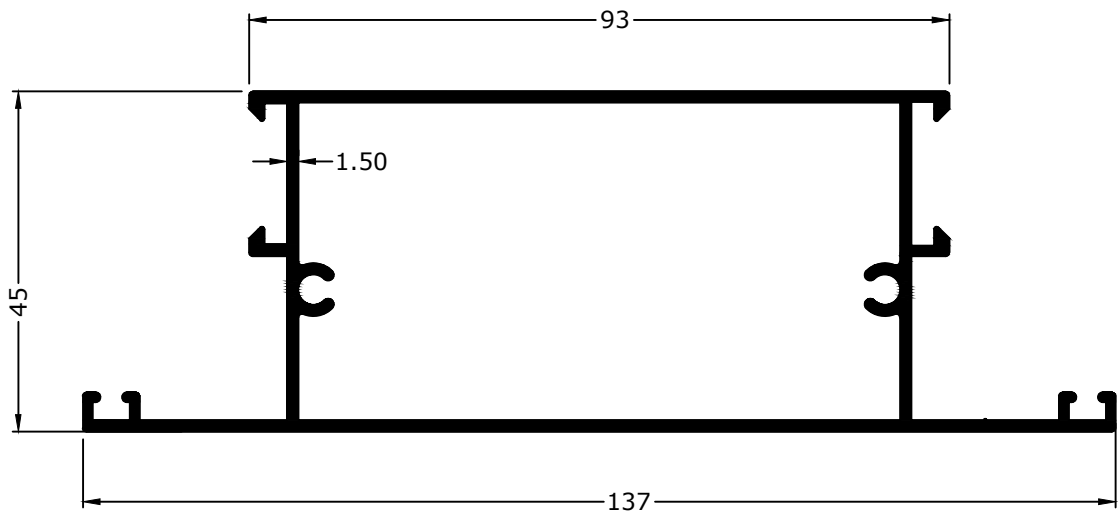
1726 1.560 KG/M
