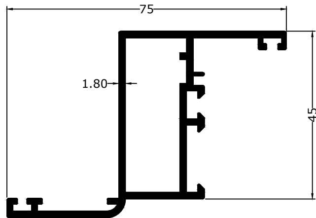
22312 1.075KG/M
