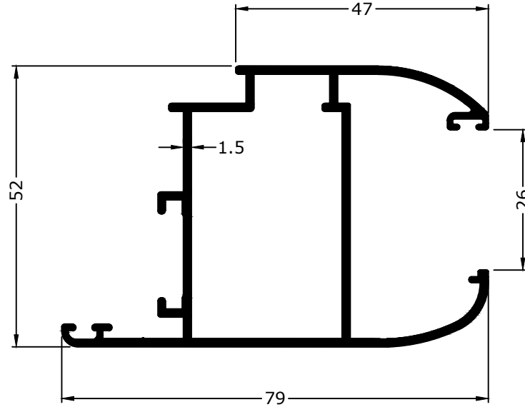
1728 1.150 KG/M
