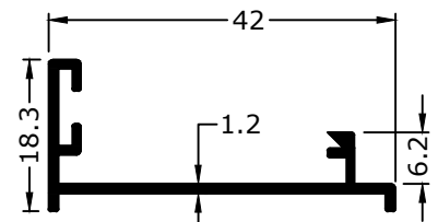
1073 0.256 KG/M
