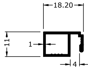
1122 0.163 KG/M
