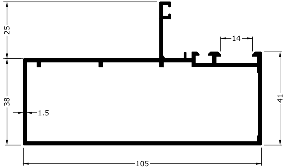
2027 1.398 KG/M
