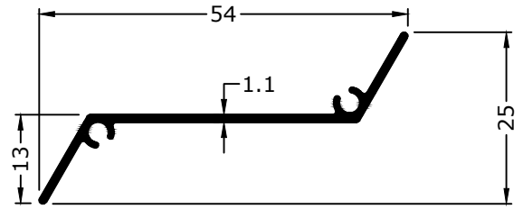
10191 0.227 KG/M
