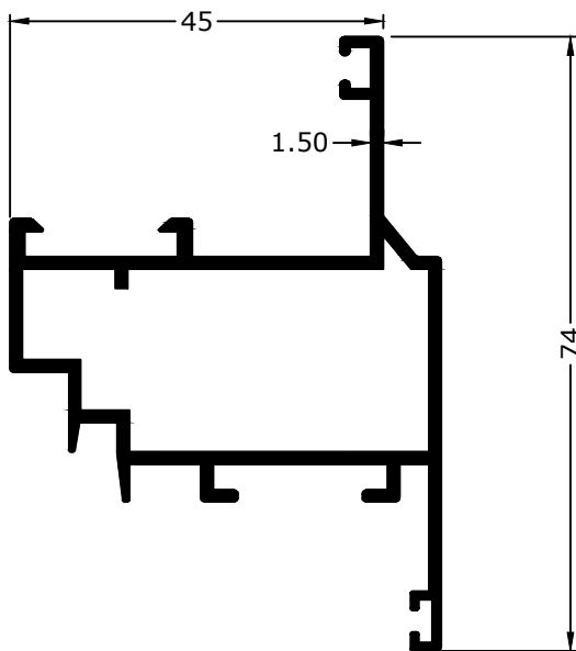
2306 1.000 KG/M
