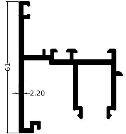
1696 1.158 KG/M
