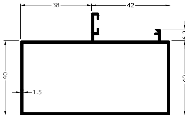
20391 1.070 KG/M
