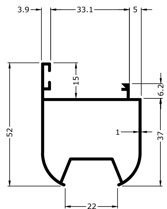
2076 0.531 KG/M
