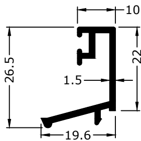
1027 0.264 KG/M
