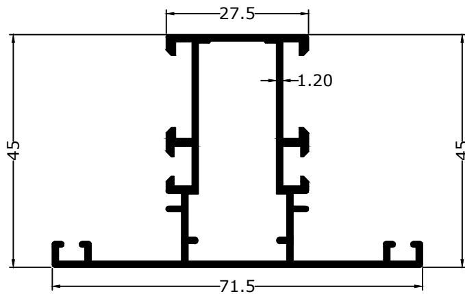
A2021 0.845 KG/M
