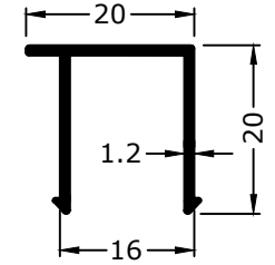
1065 0.188 KG/M
