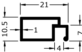
2025 0.171 KG/M
