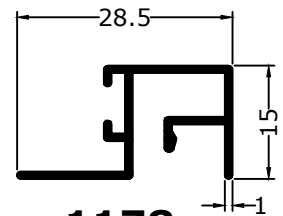
1178 0.215 KG/M
